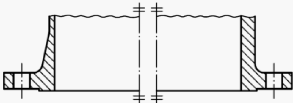
k) Type 21 Integral flange
