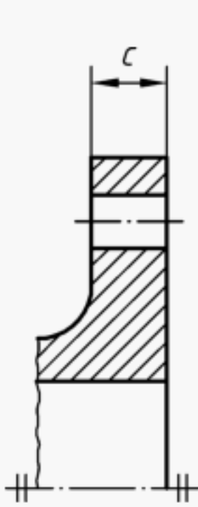
a) Type A: Flat face
