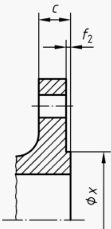
e) Type E: Spigot
