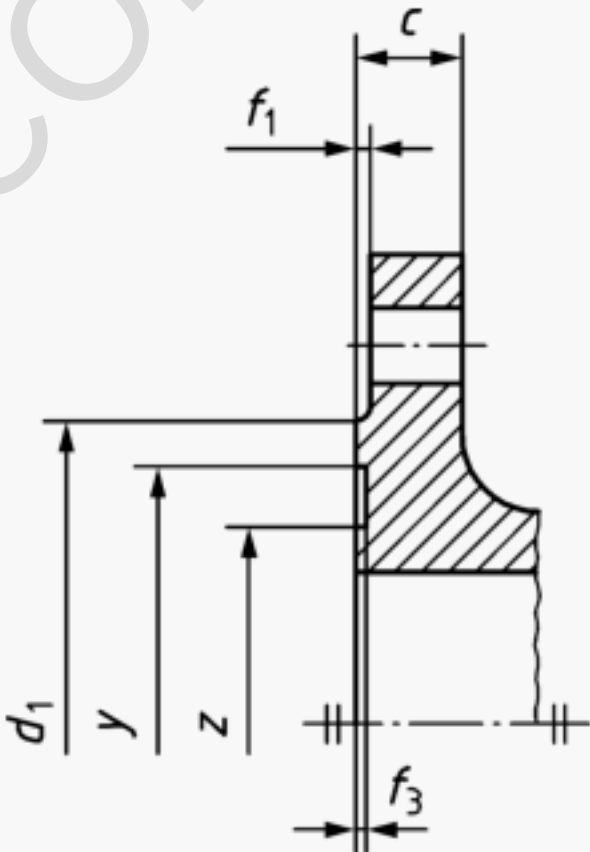
d) Type D: Groove
