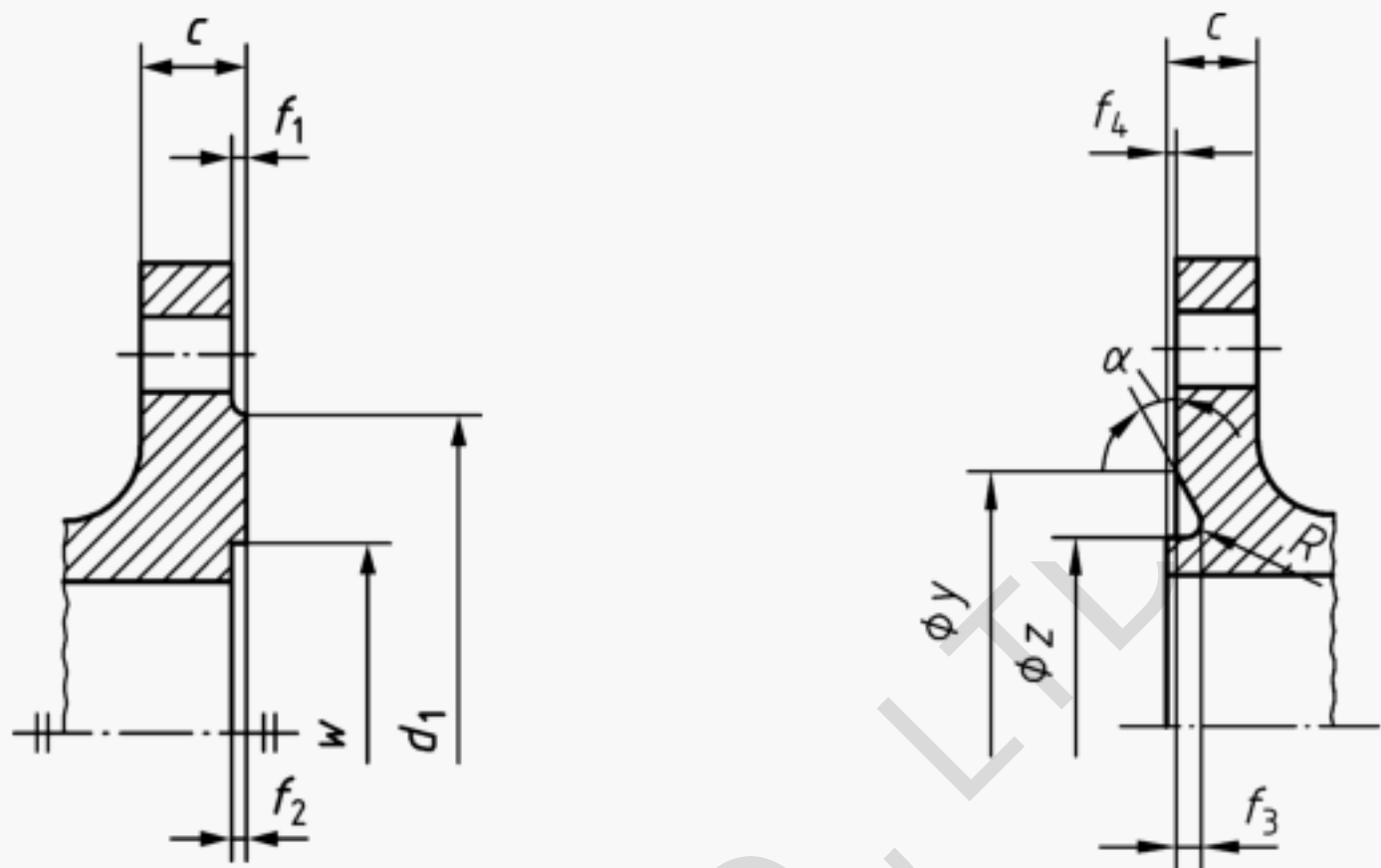
g) Type G: O-ring spigot
